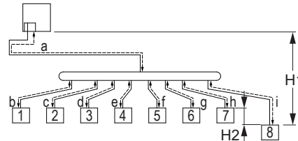
18-3 Пример 3: само в случай на рефнет колектор
