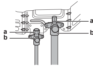
a Сервисен порт b Спирателен клапан
