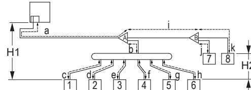
18-2 Пример 2: в случай на рефнет съединения и колектор
