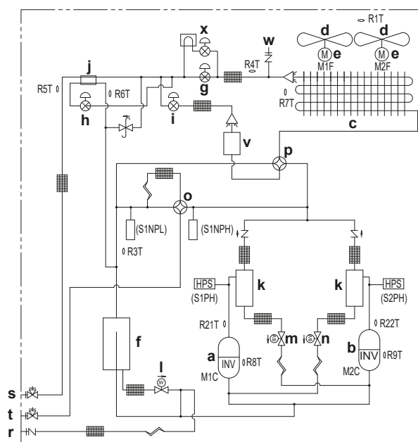
Rördragningsschema: RYYQ14~20
