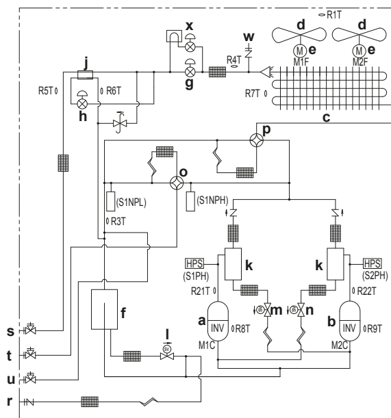
Diagram cevovoda: RYMQ14~20
