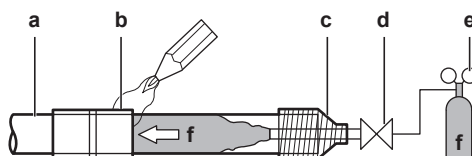
a Koelmiddelleiding b Te hardsolderen deel c Tape
