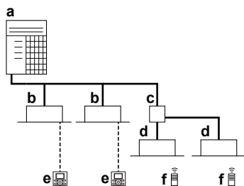
a VRV šilumos siurblio lauko blokas
