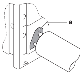
a Tömítse a nyílásokat (szürkével jelölt terület).
