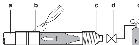
a Hűtőközegcsövek b Forrasztandó rész c Körültekercselés
