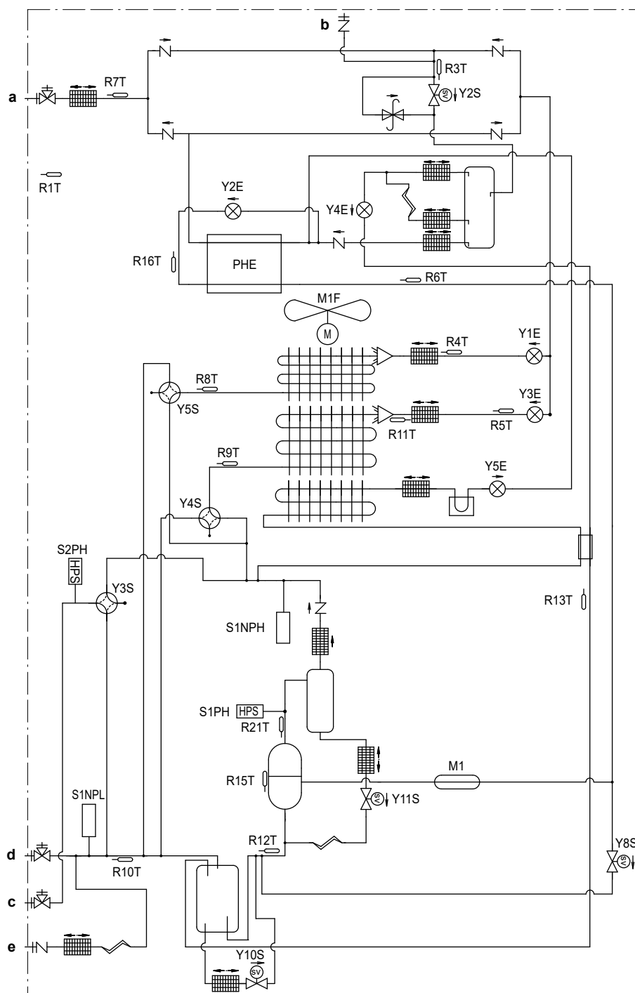
Diagram cevovoda: 5~12 HP
