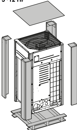
5~12 HP
