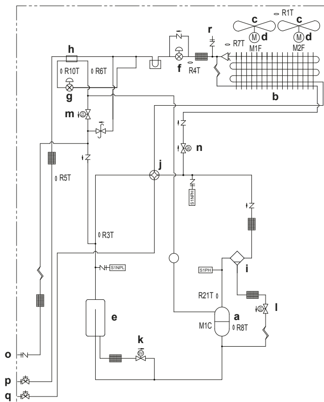
Schemat przewodów: RXMLQ8 + RXYLQ10~14
