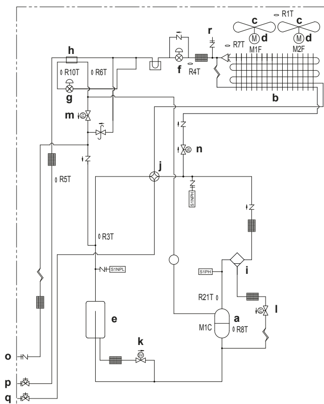
Schéma potrubí: RXMLQ8 + RXYLQ10~14
