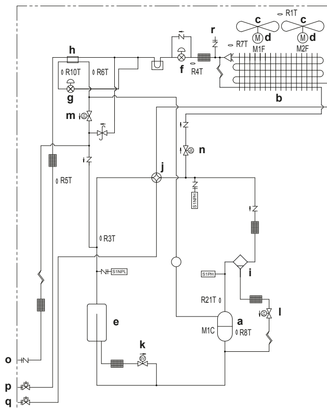
Vamzdžių schema. RXMLQ8 + RXYLQ10~14
