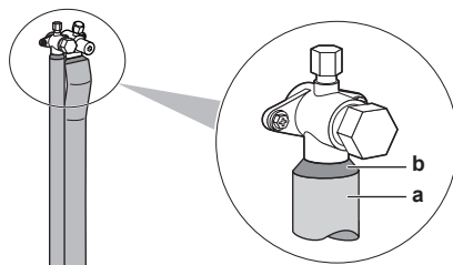
a Izoliacijos medžiaga b Kamšalas ir pan.
