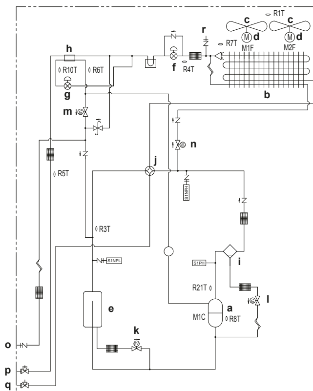
Schéma potrubí: RXMLQ8 + RXYLQ10~14
