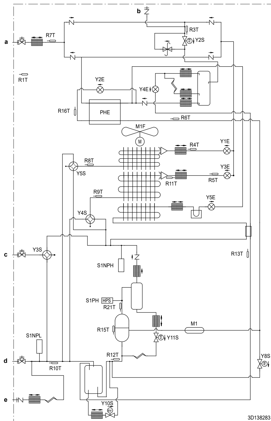
Diagram cevovoda: 5~12 HP
