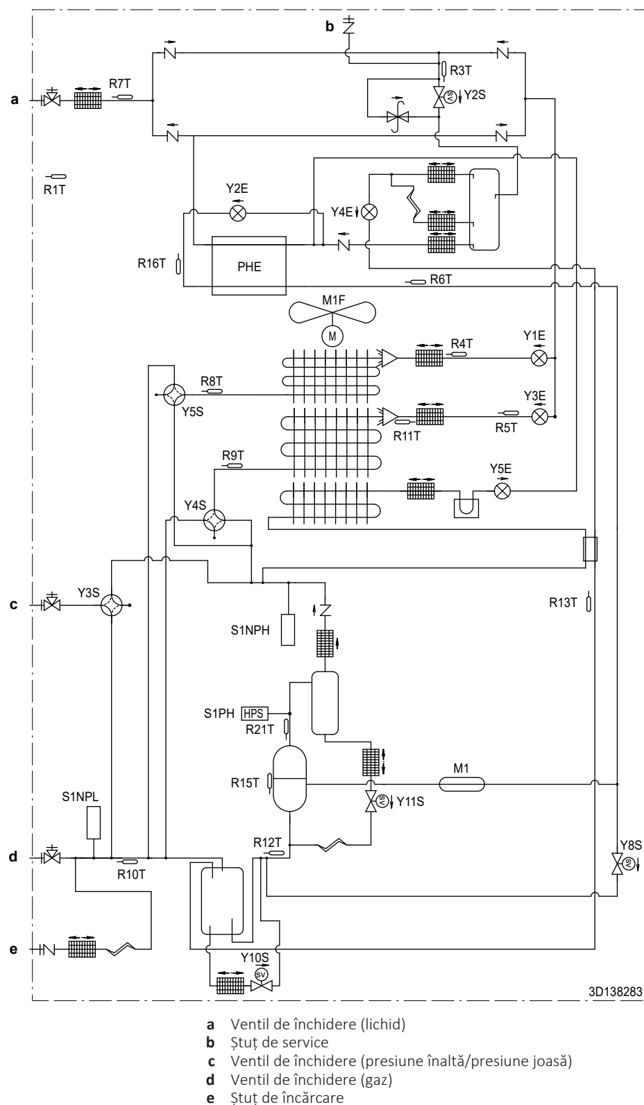
Schema tubulaturii: 5~12 HP
