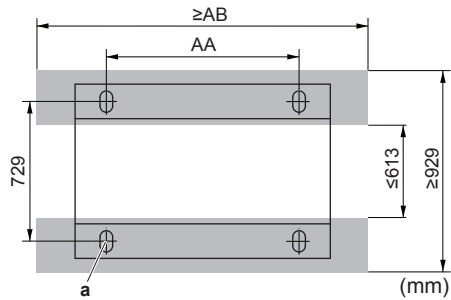
Fundație minimă a Punct de ancorare (4x)
