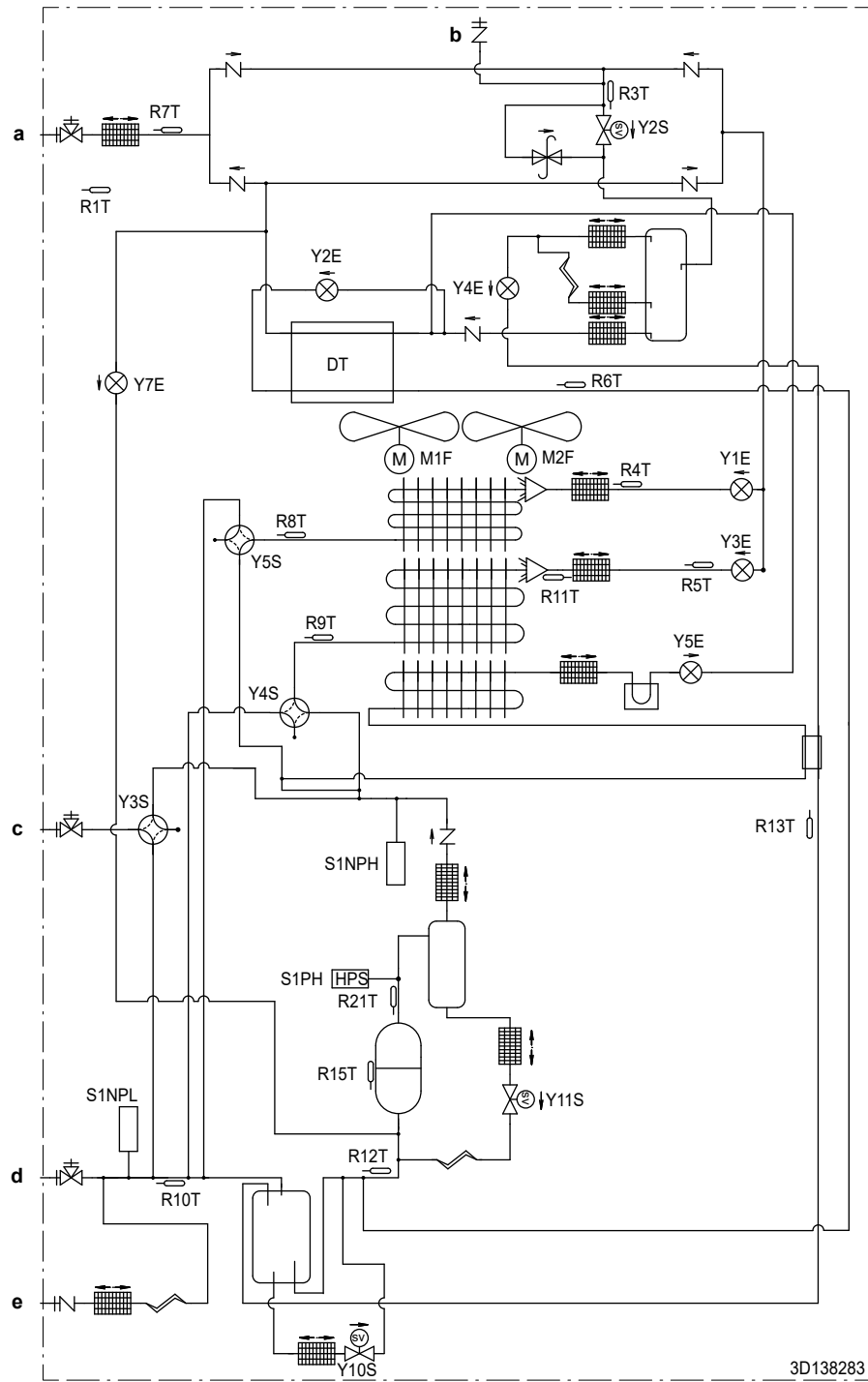
Boru hattı şeması: 14~20 HP
