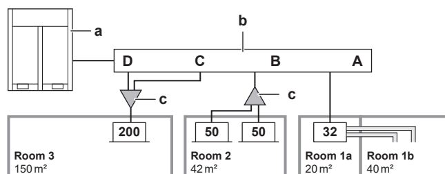
A~D Apertura dei tubi di diramazione A~D
