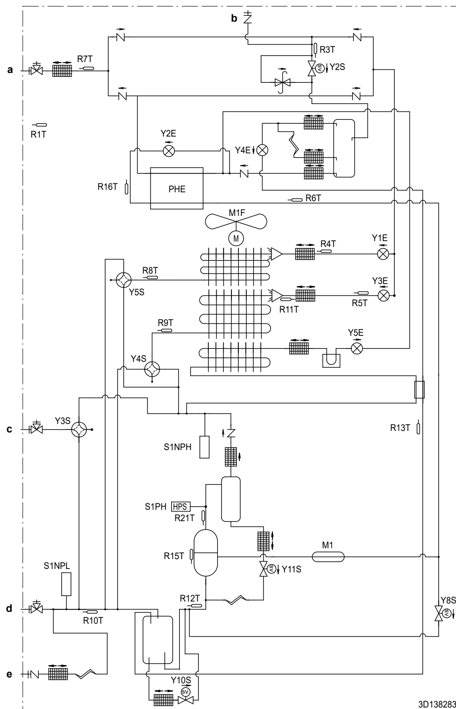
Diagrama de tubería: 5~12 HP
