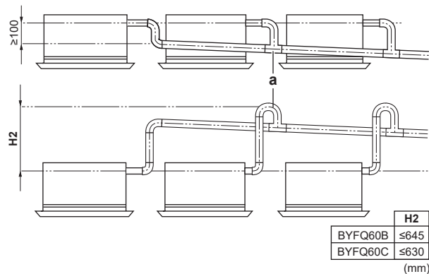
a Т-подібне з'єднання
