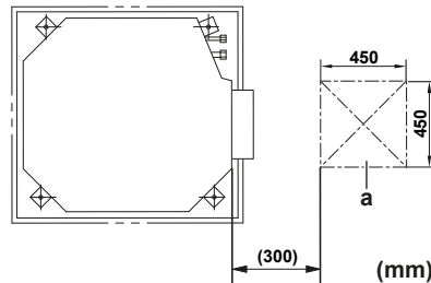
a Інспекційний отвір
