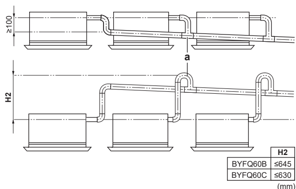
a T-stuk
