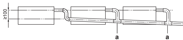
а Тройник
