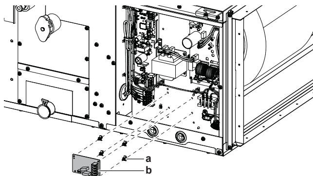
a Wspornik płytki drukowanej b Opcjonalna płytki drukowana wyjść
