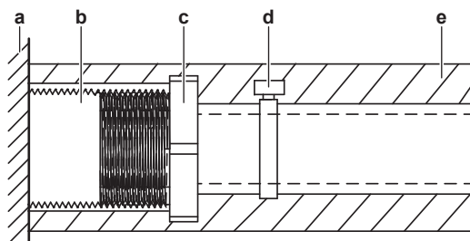
a Urządzenie wewnętrzne b Gwint wewnętrzny BSP 1" c Przejściówka (nie należy do wyposażenia) d Metalowy zacisk (nie należy do wyposażenia) e Materiał izolacyjny do przewodu odpływowego (nie należy do wyposażenia)
