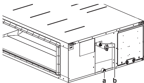
a Króciec odprowadzania skroplin b Przewody czynnika chłodniczego
