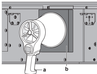
a Anemometr łopatkowy b Zestaw do podłączania kanału (EKBSDCK)
