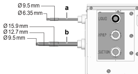
a Σωλήνας διακλάδωσης υγρού b Σωλήνας διακλάδωσης αερίου
