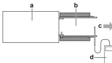
a Μονάδα BS b Αεραγωγός εξόδου αέρα c Κατεύθυνση ροής αέρα d Ανεμόμετρο θερμού καλωδίου
