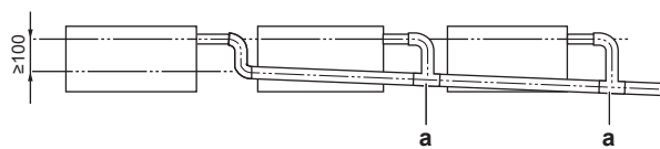
a T-stykke
