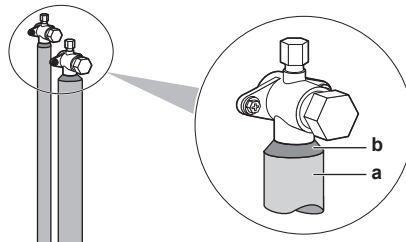
a Isolatiemateriaal b Afdichtingsmateriaal, enz.
