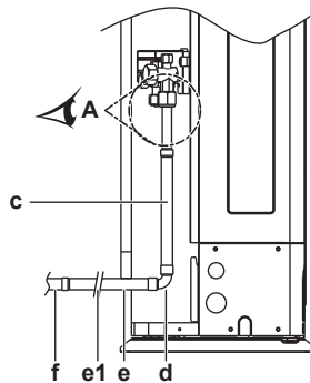
Mogelijkheid 3: Naar de zijkant
