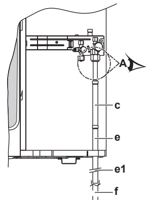
Mogelijkheid 4: Naar onder
