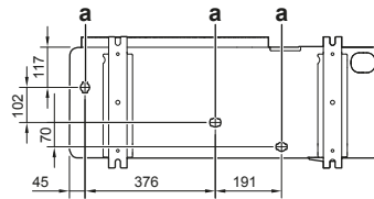
a Fori di scolo
