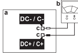
a لوحة الدوائر المطبوعة الرئيسية b المقياس المتعدد c نقاط القياس
