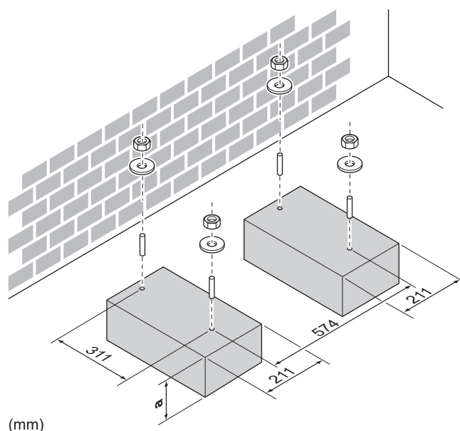
a 100 mm over forventet højde på snelag
