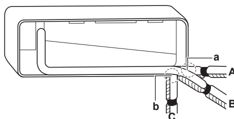
A Kreisās puses cauruļvads B Cauruļvads pa kreisi aizmugurē C Cauruļvads pa kreisi apakšā a Šeit izņemiet cauruļu atveres vāciņu cauruļvadā kreisajā pusē b Šeit izņemiet cauruļu atveres vāciņu cauruļvadā aizmugurē apakšā pa kreisi
