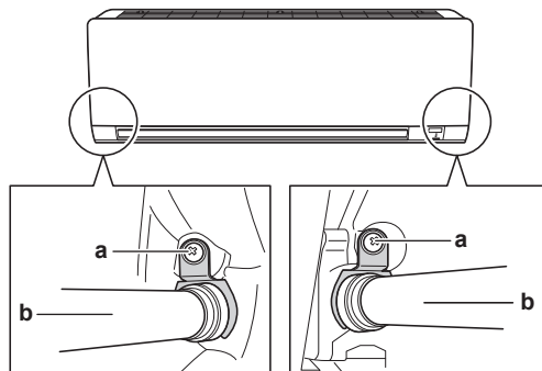
a Винт за закрепване на изолация b Дренажен маркуч
