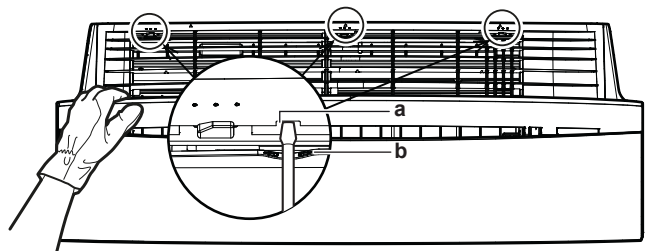
a Ranura b Hendidura en forma de media luna
