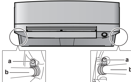
a Tornillo de fijación del aislamiento b Manguera de drenaje
