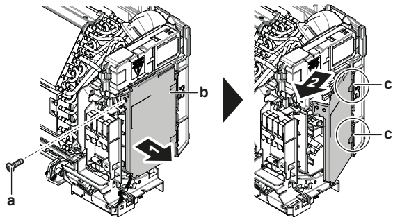
a Tornillo b Caja de cableado eléctrico c Gancho trasero
