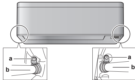
a Yalıtım tespit vidası b Drenaj hortumu
