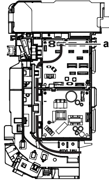
a S21 konektörü
