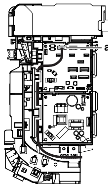
a S21-koblingsstykke
