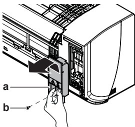
a Кришка люка для обслуговування
