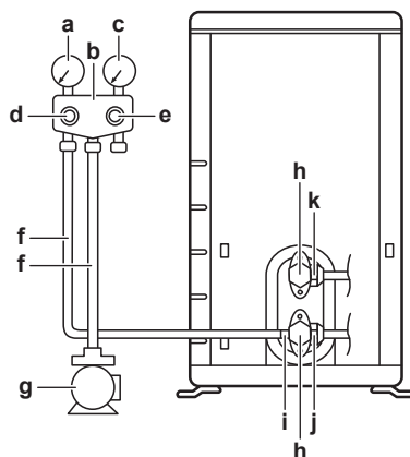
a Lavtrykksmåler
