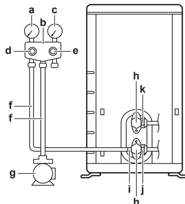
a Lavtrykksmåler
