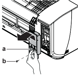
a Servis kapağı b Servis kapağı vidası
