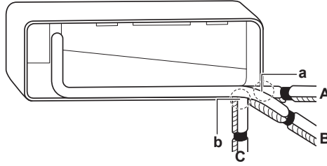
A Sol yandan boru bağlantısı B Sol arkadan boru bağlantısı C Sol alttan boru bağlantısı a Sol yandan boru bağlantısı için boru portu kapağını buradan çıkarın b Sol alttan boru bağlantısı için boru portu kapağını buradan çıkarın
