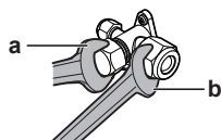
a Француски клуч b Моментен клуч
