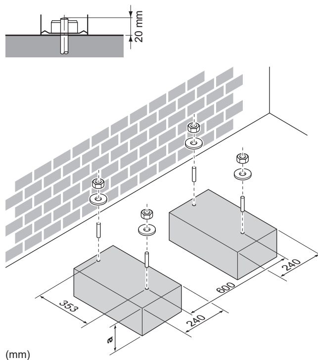
a 100 mm deasupra nivelului anticipat al zăpezii
