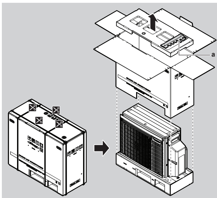
a Звукоизолационна част
