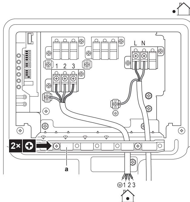
a Dispositivo de retención de los cables
