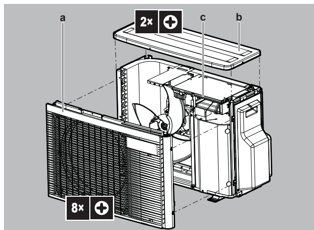
a Предна плоча b Горна плоча c S99 конектор
