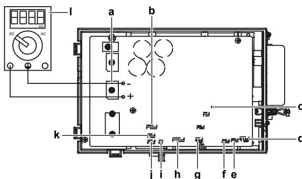
a DB1 диоден мост
