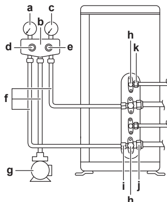
a Измерител на ниско налягане
