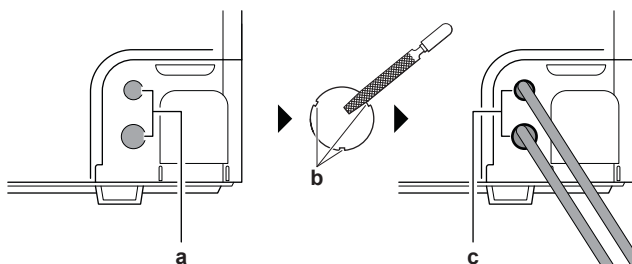
a Выбивное отверстие b Заусенец
