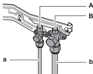
A Sulkuventtiili (neste) B Sulkuventtiili (kaasu) a Nesteputki b Kaasuputki
