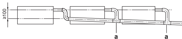
a T veida savienojums
