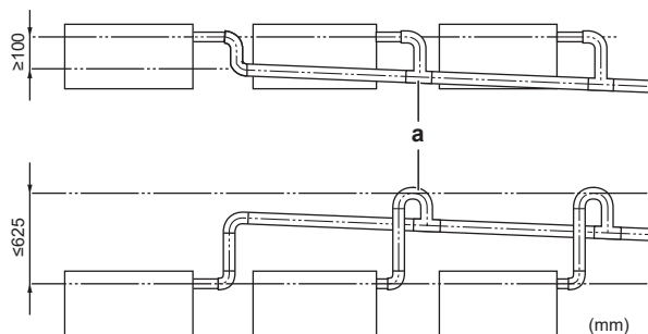
a T-koppling
